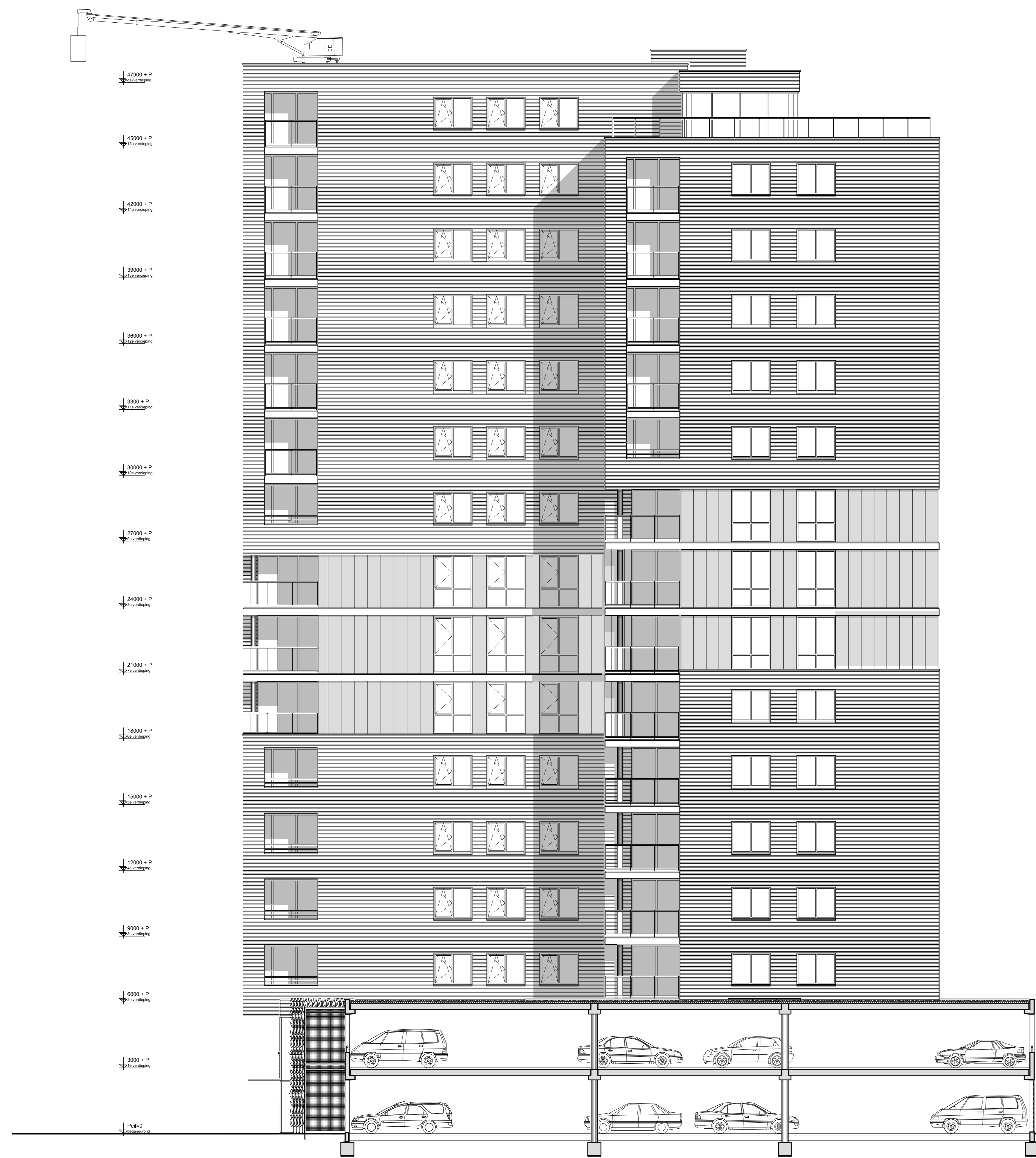
NOORDWEST GEVEL
