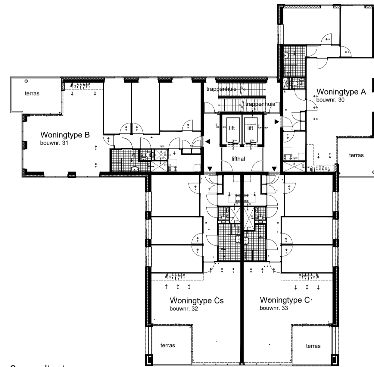
9e verdieping
