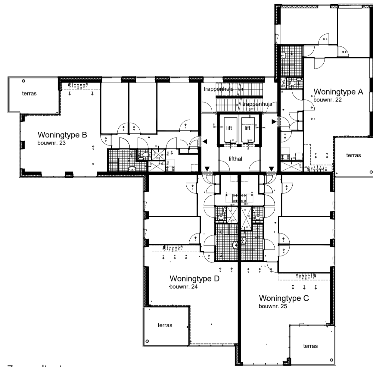
7e verdieping
