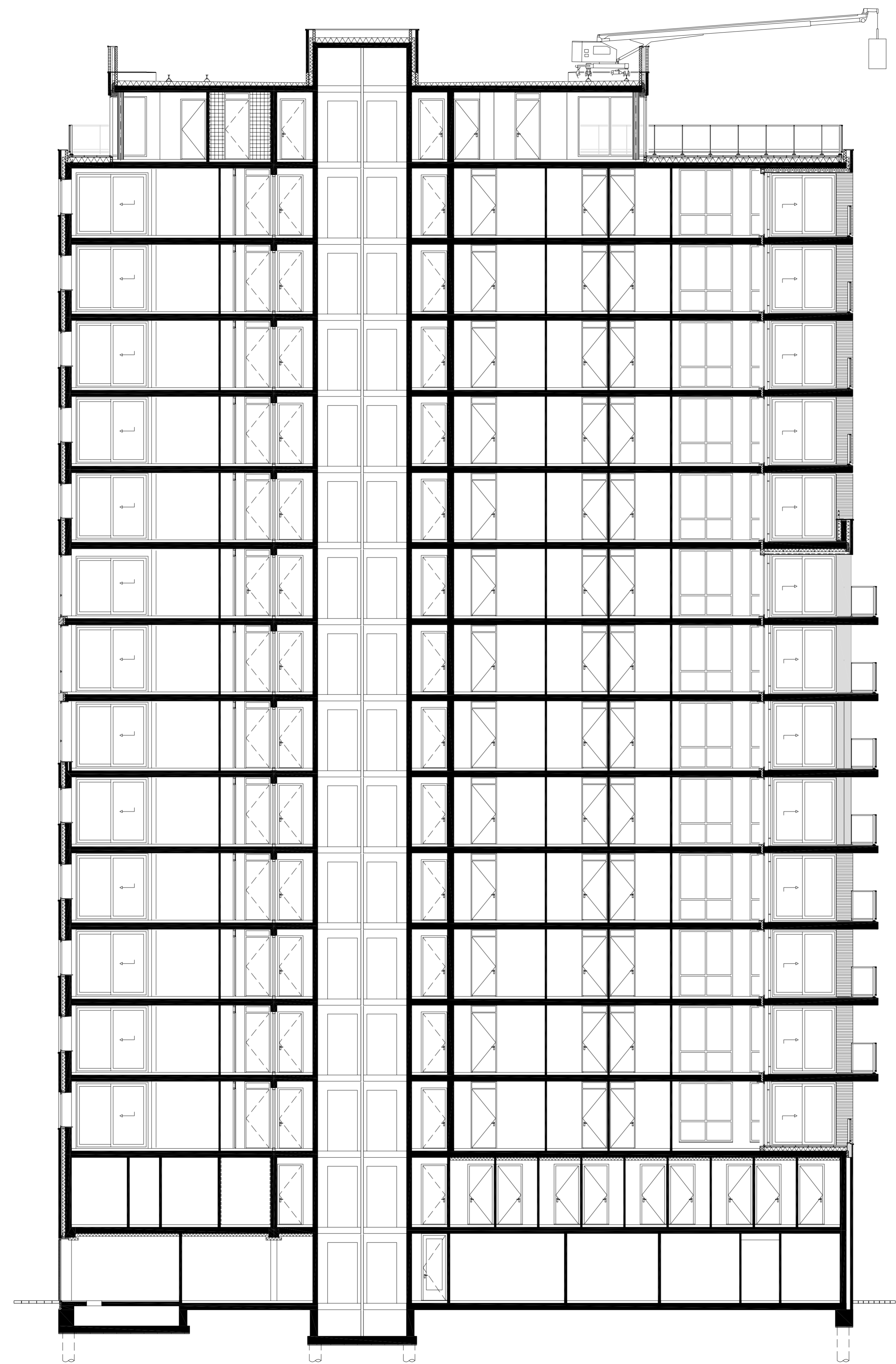
DOORSNEDE
